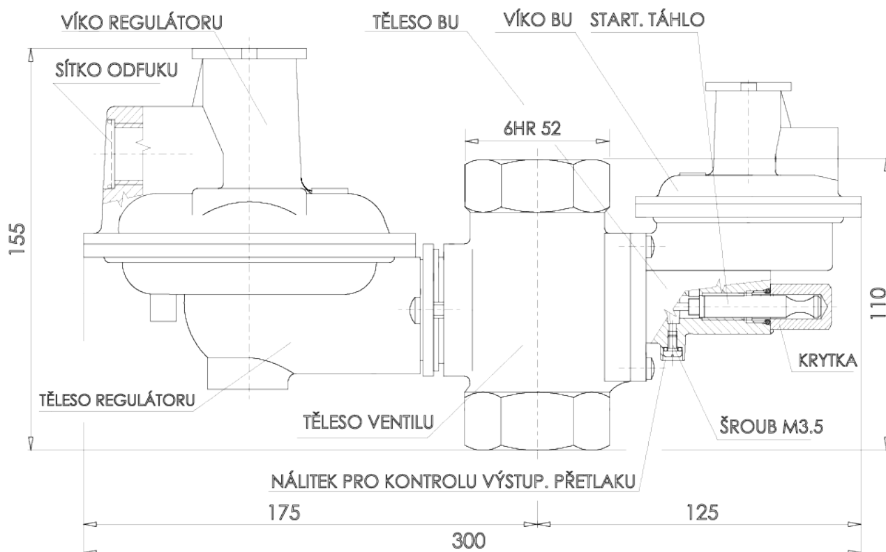
Kresba 1: Schéma regulátoru RP – 6/10
