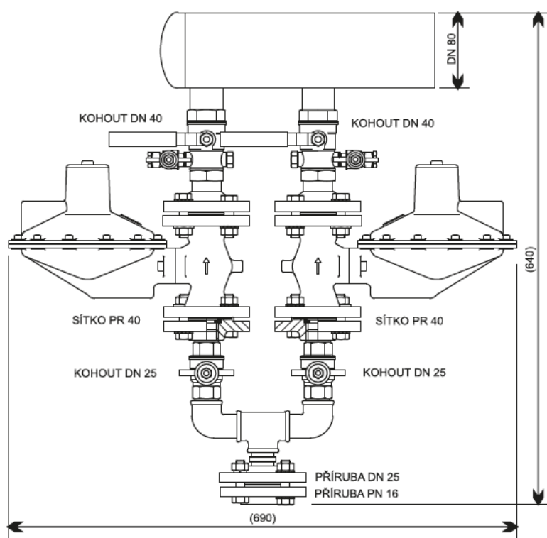
Kresba 3: Schéma dvojité regulační soupravy SS2 Alz-6U
