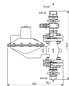
Kresba 16: Regulátor ALz-6U v závitovém provedení
