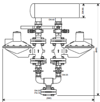
Kresba 17: Dvojitá řada v přírubovém provedení
