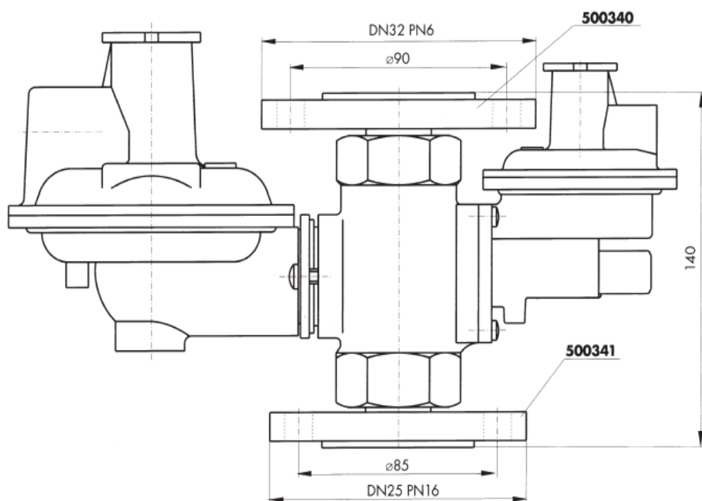
Kresba 20: Regulátor v přírubovém provedení
