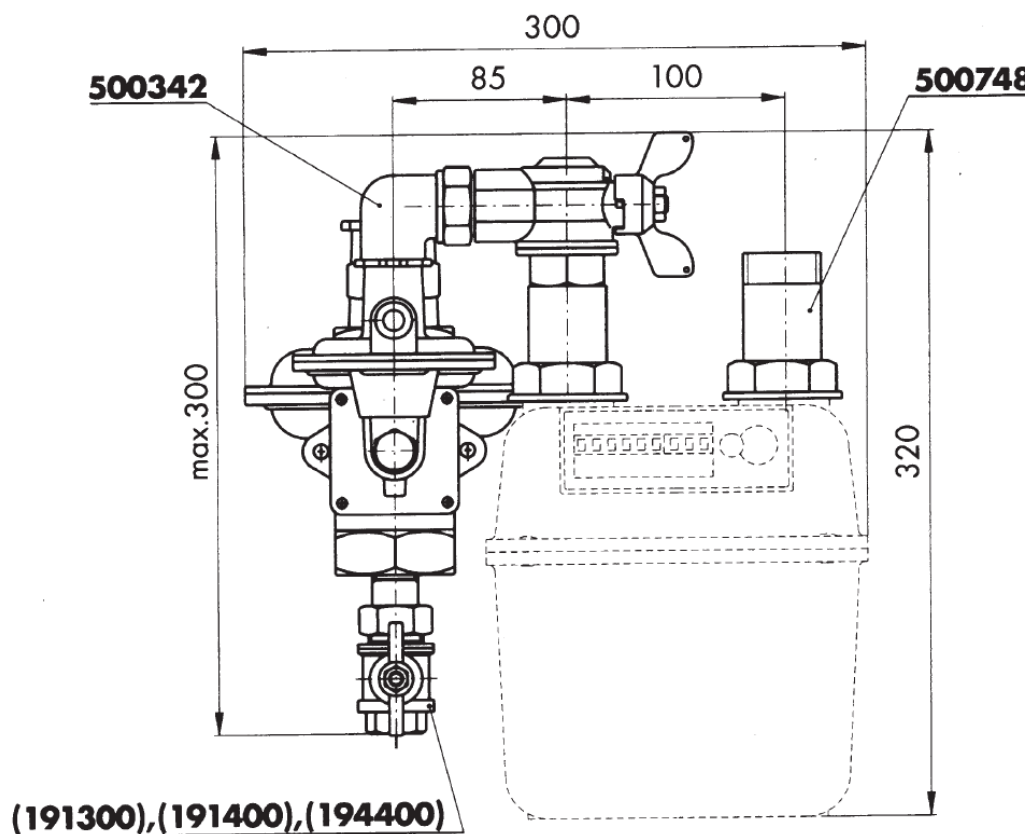
Kresba 12: Úzká skříň – regulátor otočen o 90°, plynoměr s roztečí 100 mm
