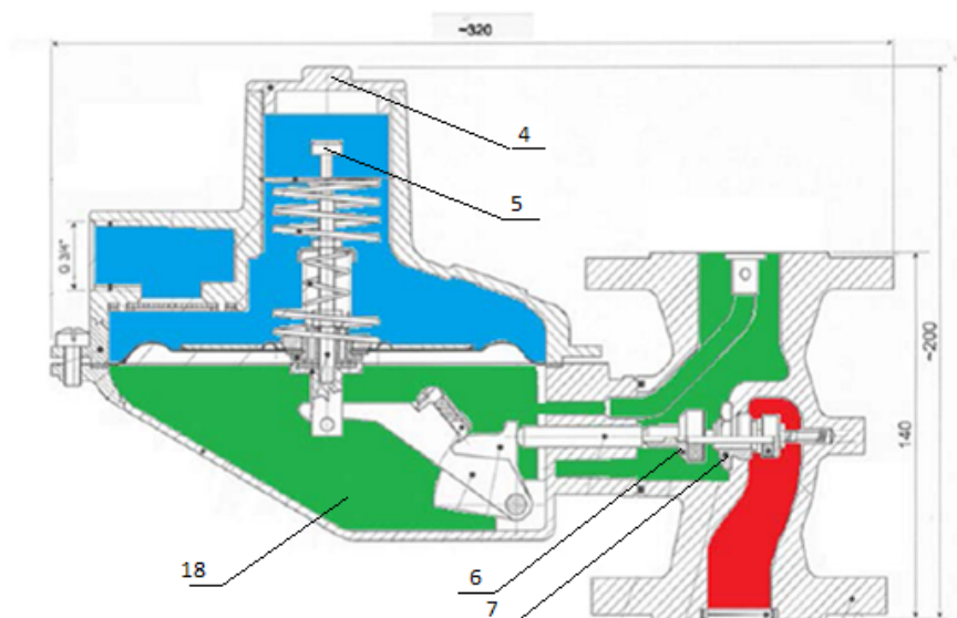
Kresba 8: Funkční schéma regulátoru ALz-6U
