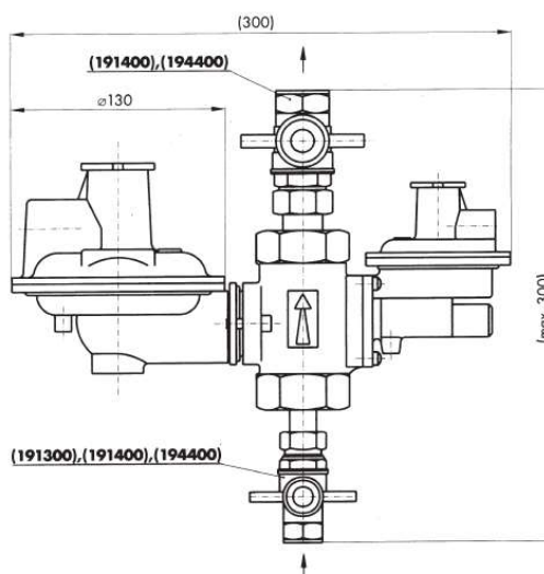
Obrázek 11: Plynoměrná skříň pro domovní regulátory RP
