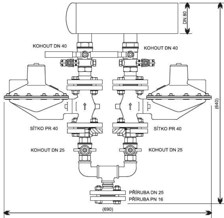
Obrázek 3: Schéma dvojité regulační soupravy SS2 Alz-6U
