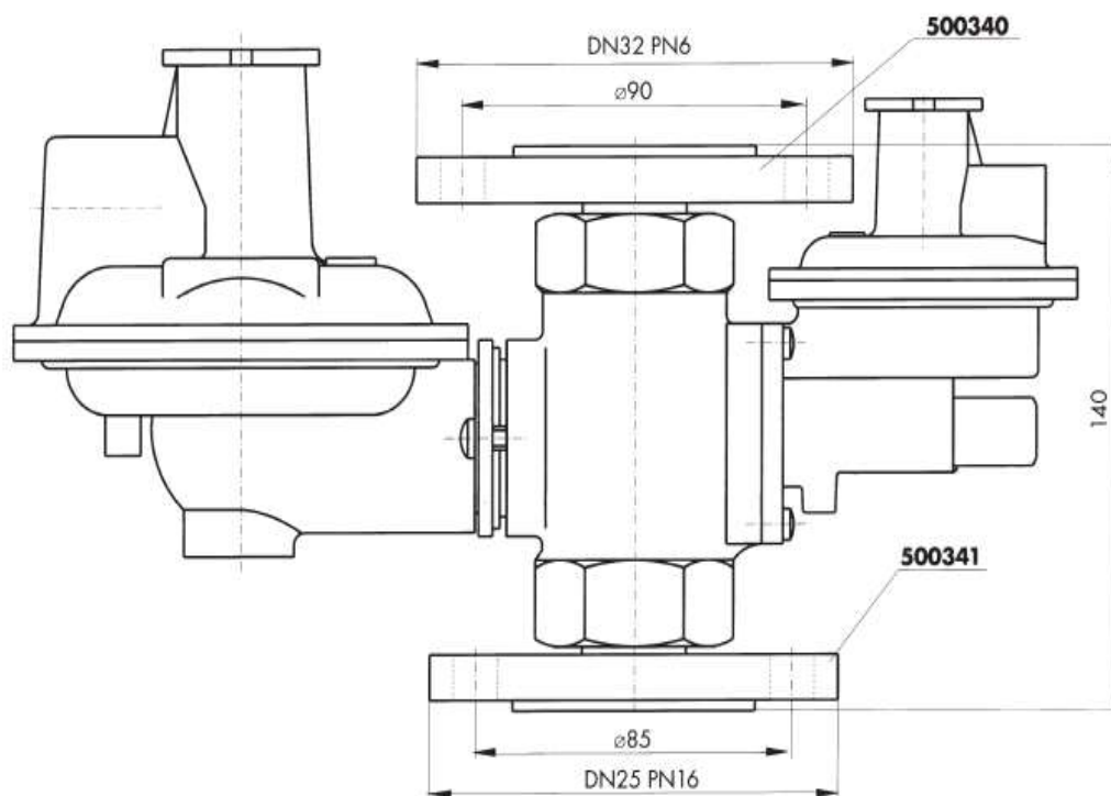
Obrázek 20: Regulátor v přírubovém provedení
