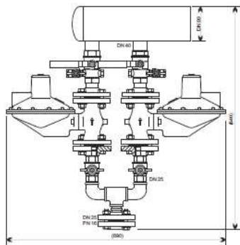
Obrázek 17: Dvojitá řada v přírubovém provedení
